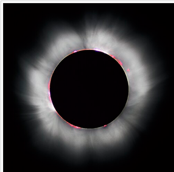
Sonnenfinsternis 1999
